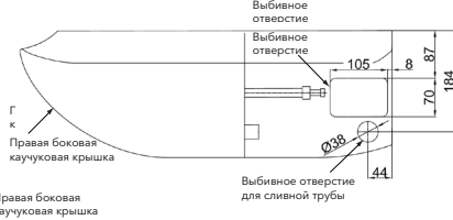
(В) Труба со стороны правой крышки
