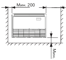
Для потолочной установки
