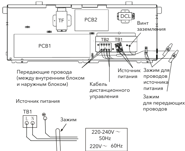
Передающий провод
