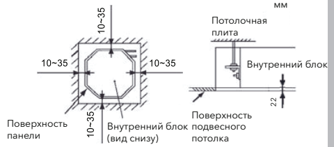
(а) Потолочный монтаж с панелью
