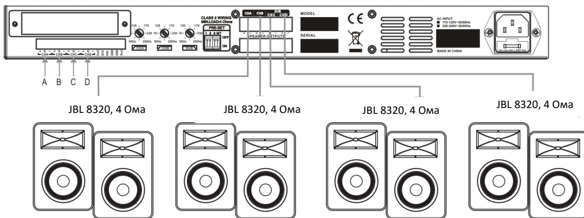
Режим 1. Все каналы стерео
