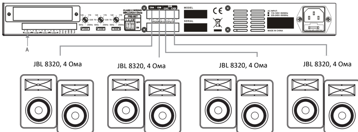
Режим 2. Все каналы параллельны
