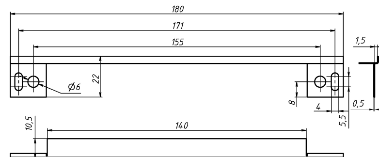
Рисунок 7 – Планка декоративная
