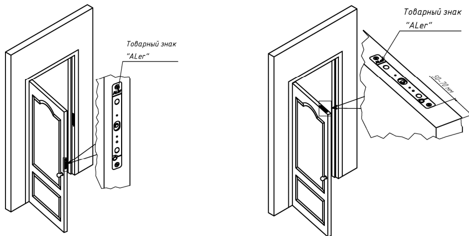
Рисунок 2 – Установка замка в вертикальном варианте
