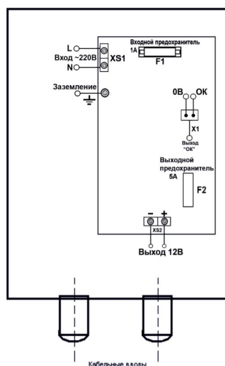
Крепление на DIN-рейку (рис.2)
