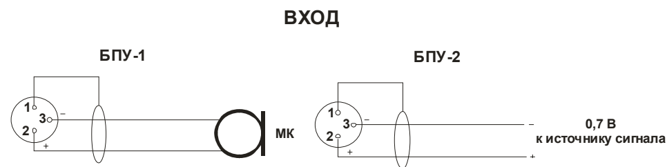
Схема подключения
