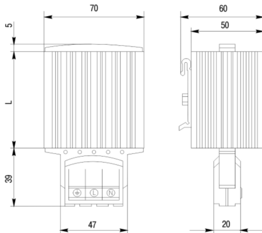
Рисунок 1 Габаритные размеры обогревателей
