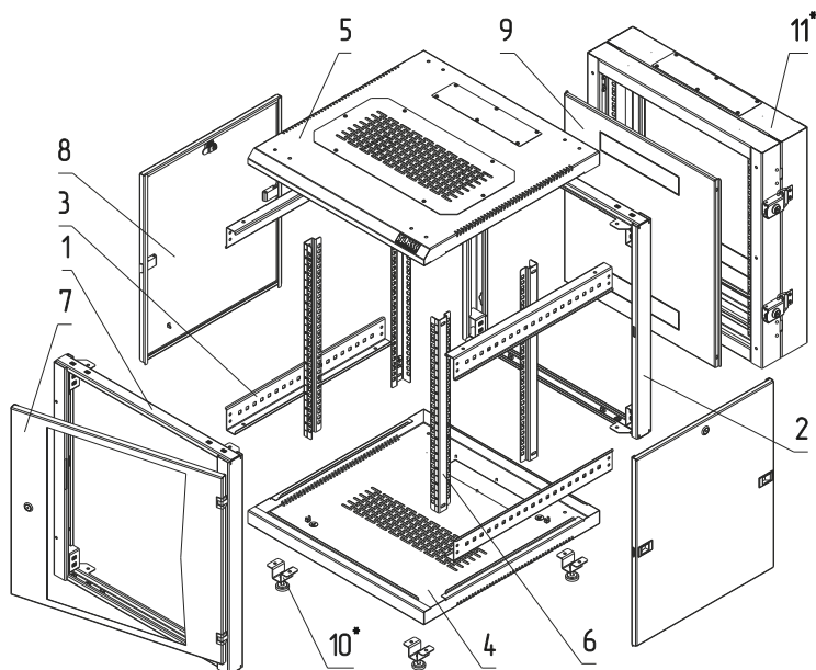
TWC-126060-R-G-GY Настенный односекционный шкаф 19", 12U, Разнесенный вид
