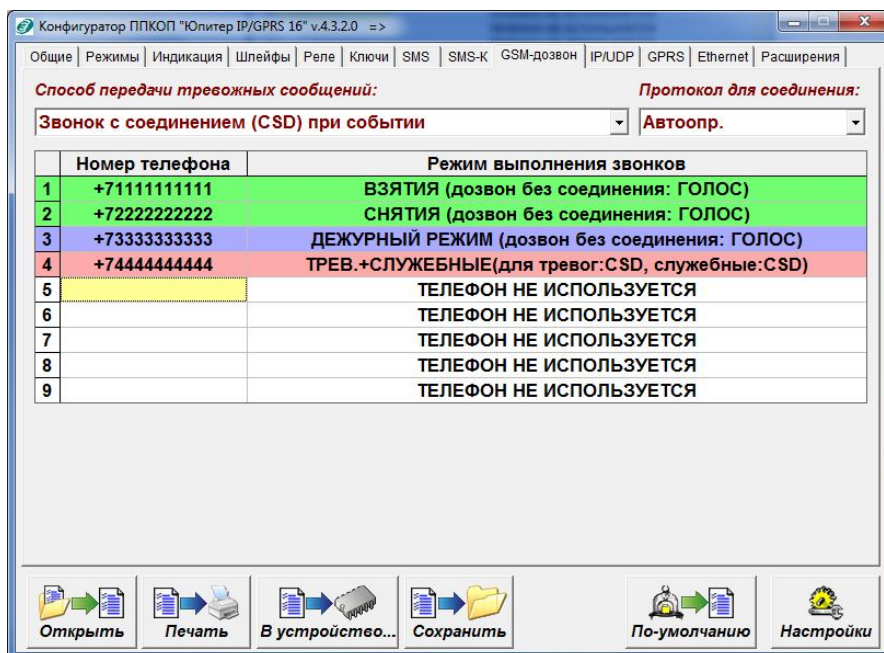
Рисунок 3.1. Настройка номеров для дозвона
