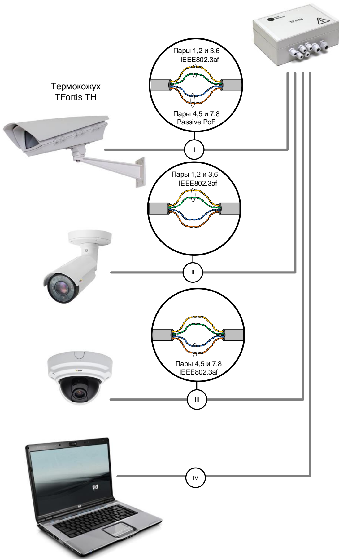
Рис. 2.3. Схема питания по PoE для разных случаев
