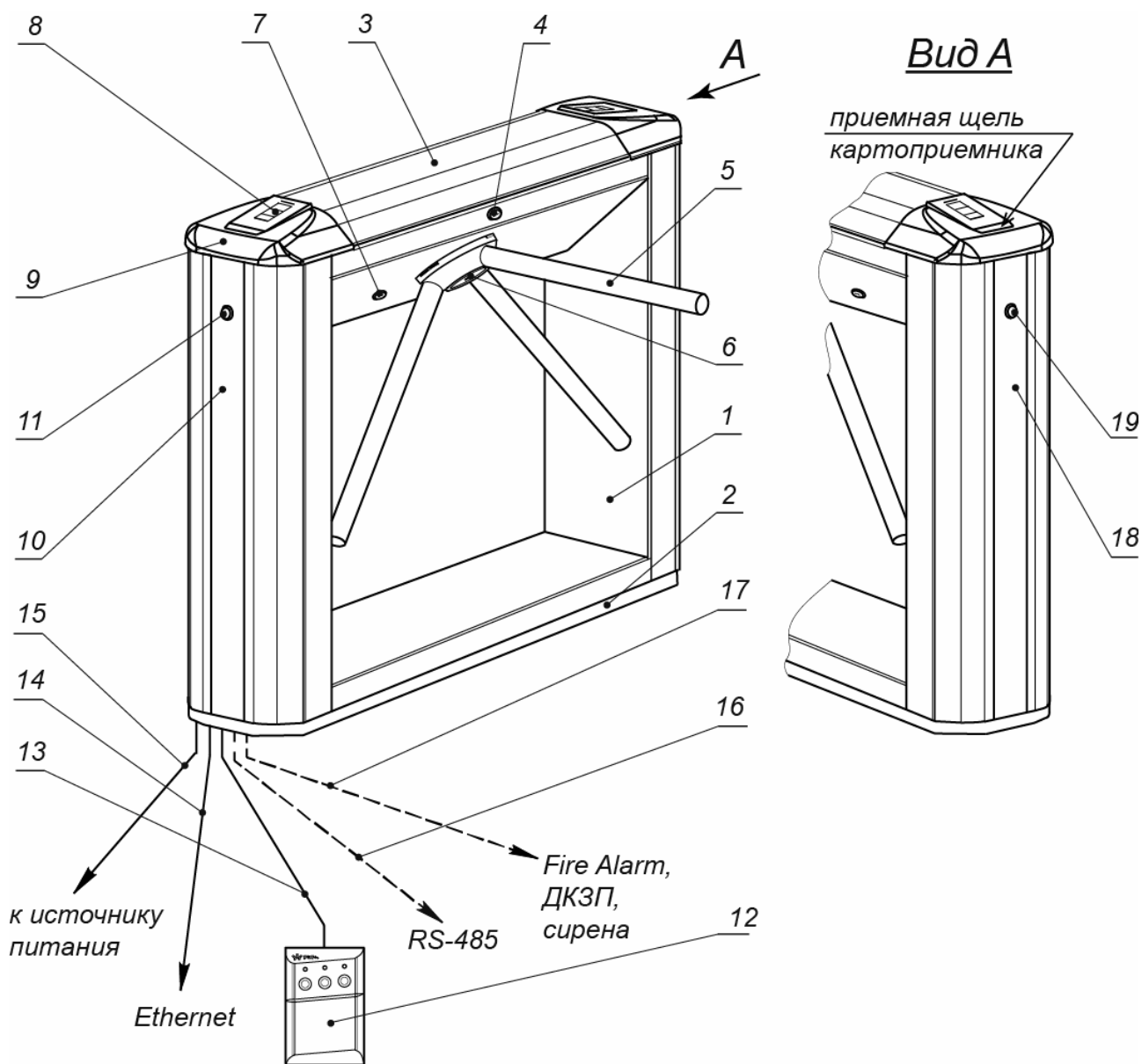
Рисунок 1. Устройство ЭП
