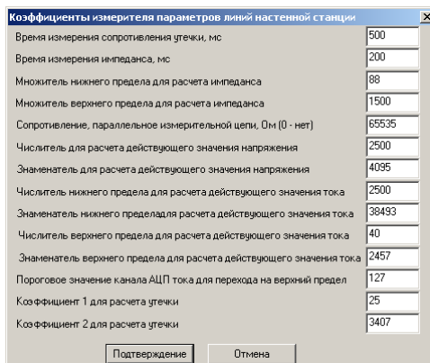
Рисунок 7.7. Диалоговое окно настройки коэффициентов измерителя параметров линий.
