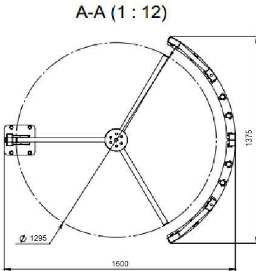
Рис. 6. Установочные размеры
