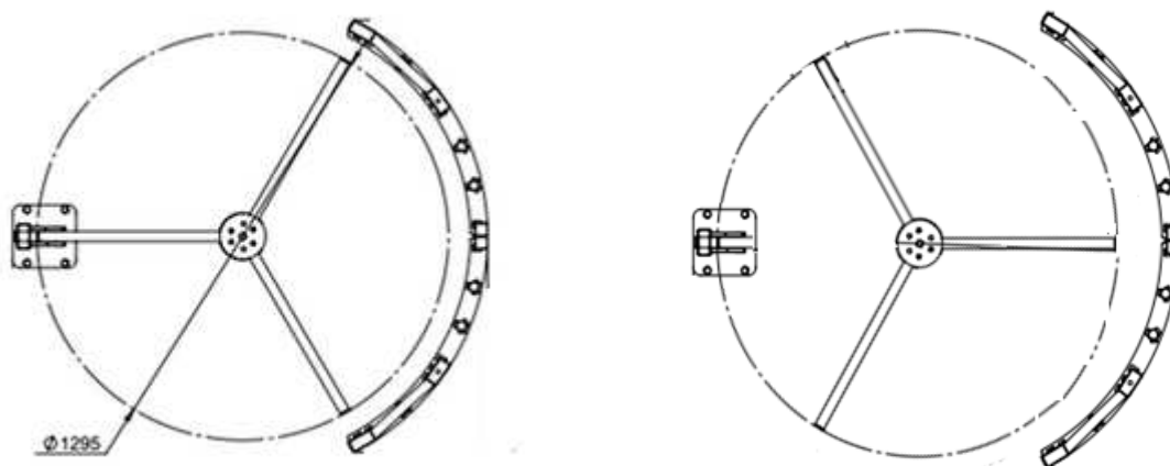
Рис. 1. Исходное положение створок турникета (вид сверху) для шлюзового режима работы
