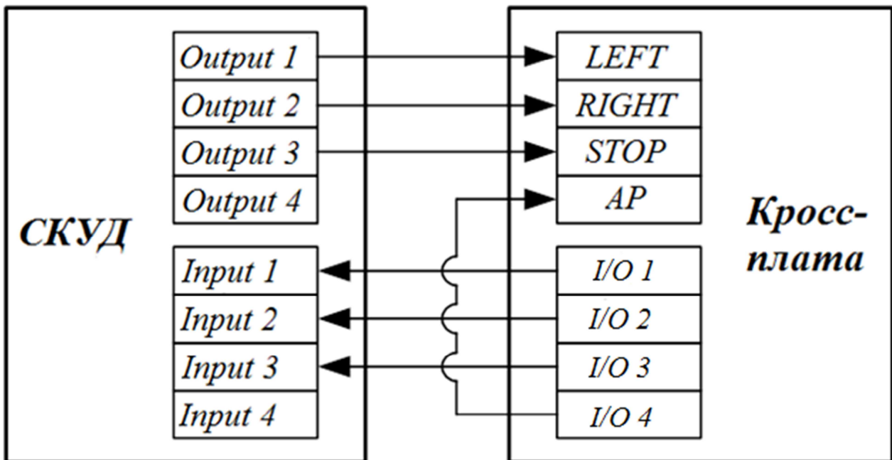
Рис. 19. Схема подключения пульта управления к контроллеру СКУД
