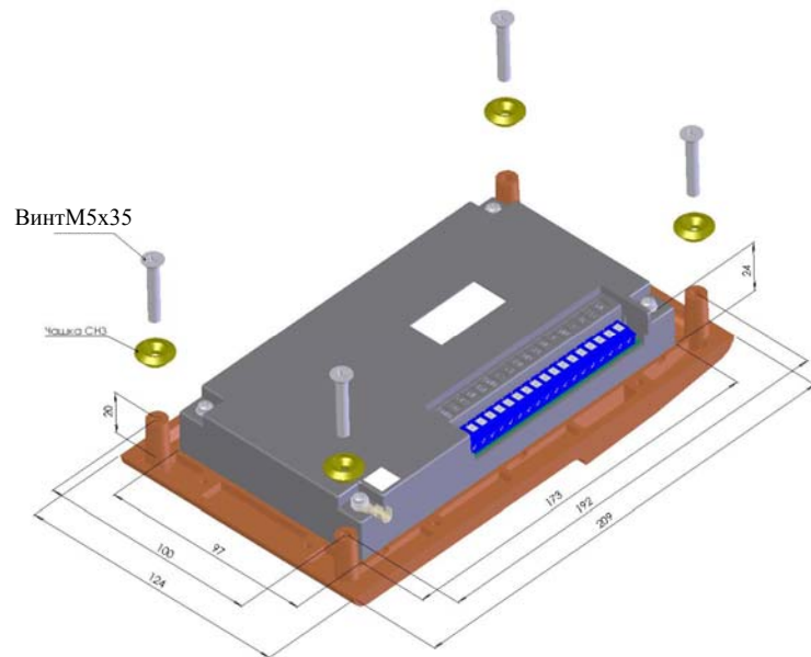
Рис.1. Внешний вид устройства с комплектом крепления КМ2
