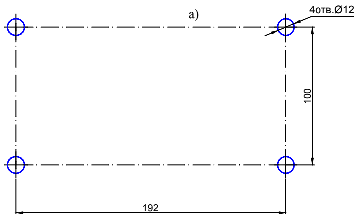
Рис.2. Разметка под установку изделия: а) снаружи; б) изнутри.
