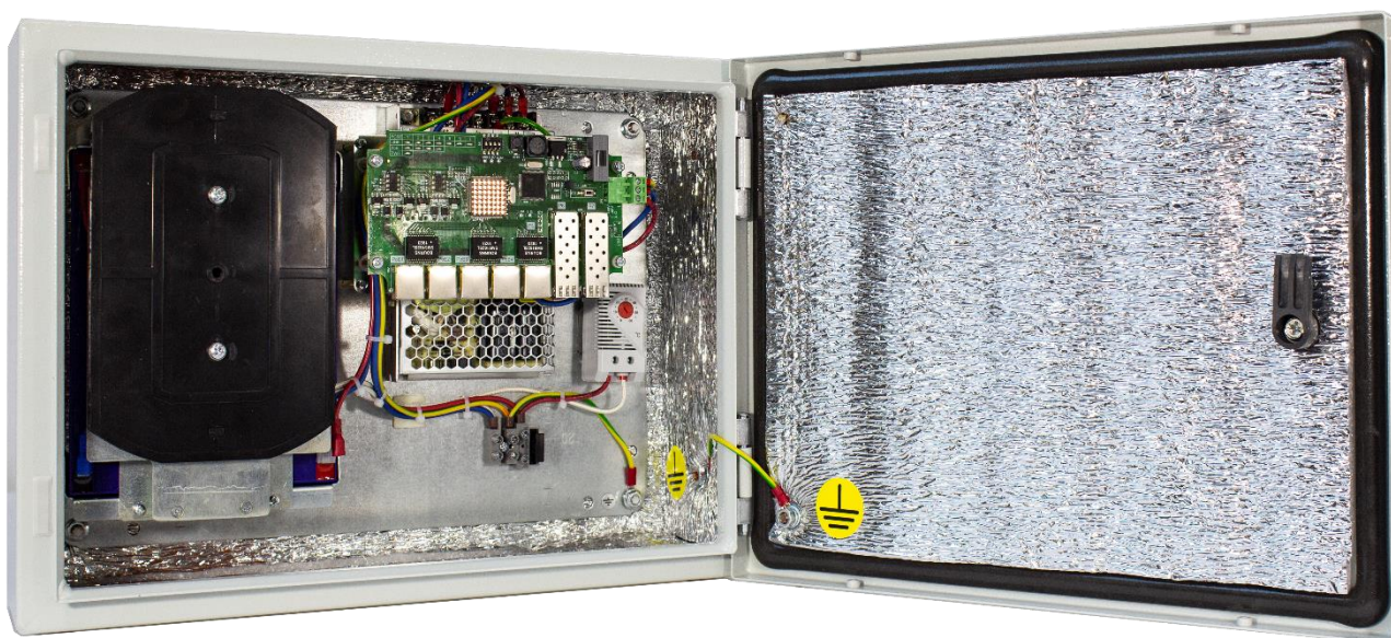
Рисунок 4. Вид изнутри
