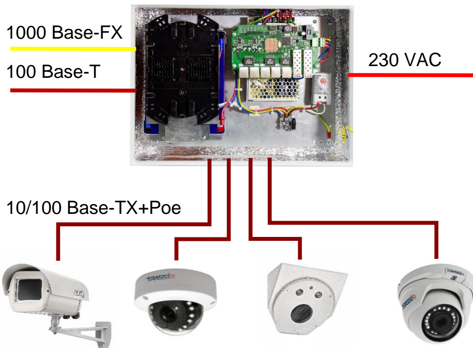
Рисунок 2. Типовая схемы подключения коммутатора по одному оптическому и одному медному кабелю.
