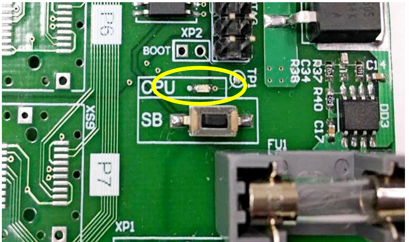
Рисунок 12. Расположение элементов индикации и настройки на плате коммутатора
