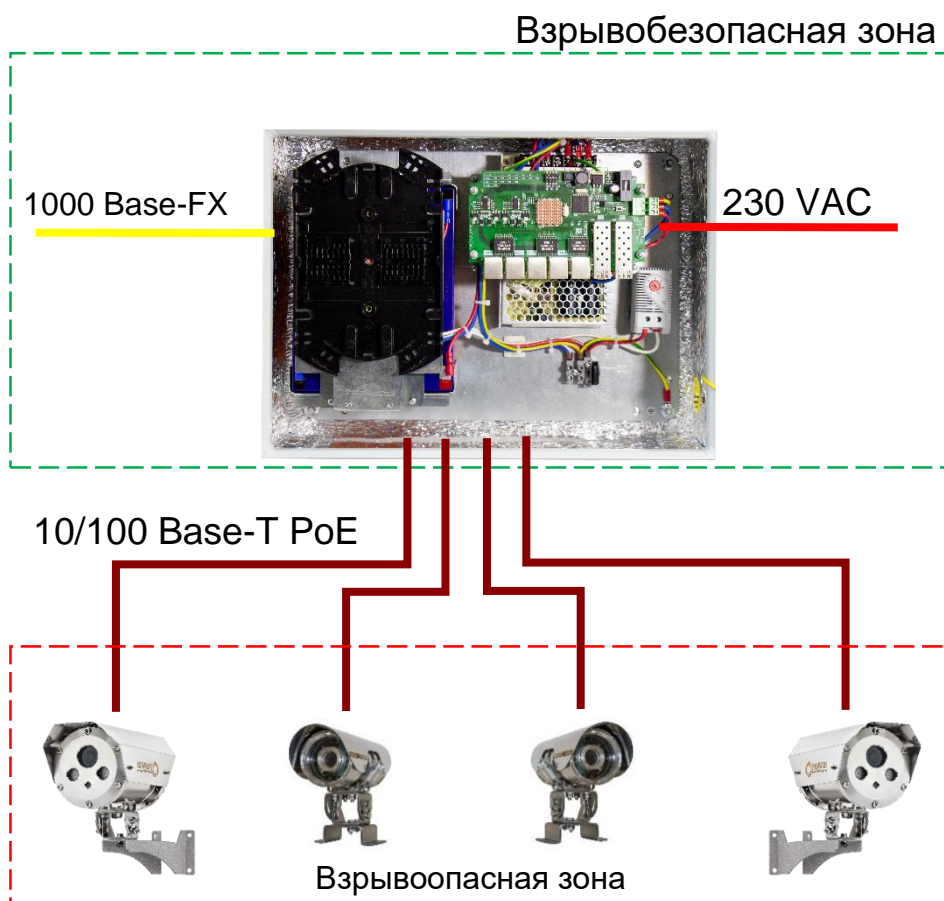
Рисунок 1. Типовая схема подключения коммутатора по одному оптическому кабелю.
