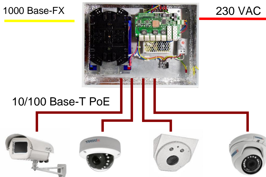
Рисунок 1. Типовая схема подключения коммутатора по одному оптическому кабелю.
