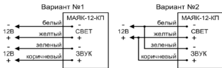
Рис.1 Схема подключения.
